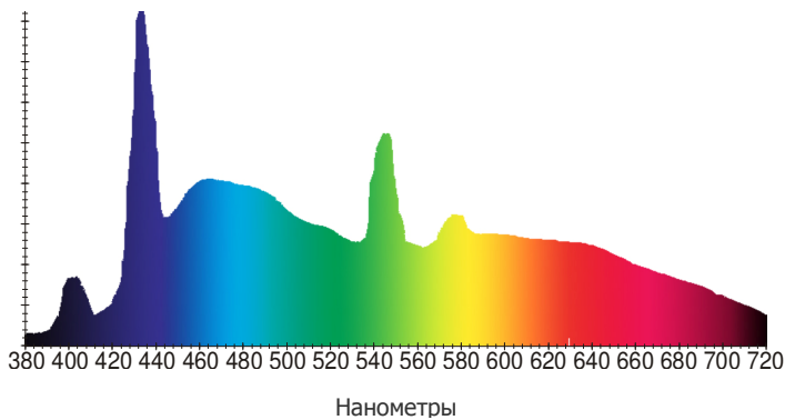
Разряд с ртутными парами при низком давлении
