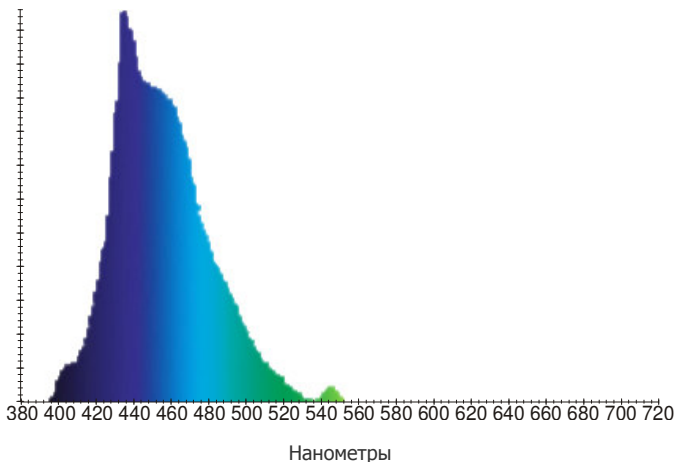
Спектральное распределение
