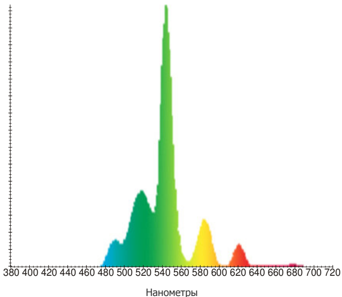
Разряд с ртутными парами при низком давлении
