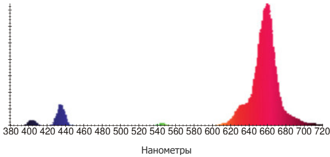
Разряд с ртутными парами при низком давлении
