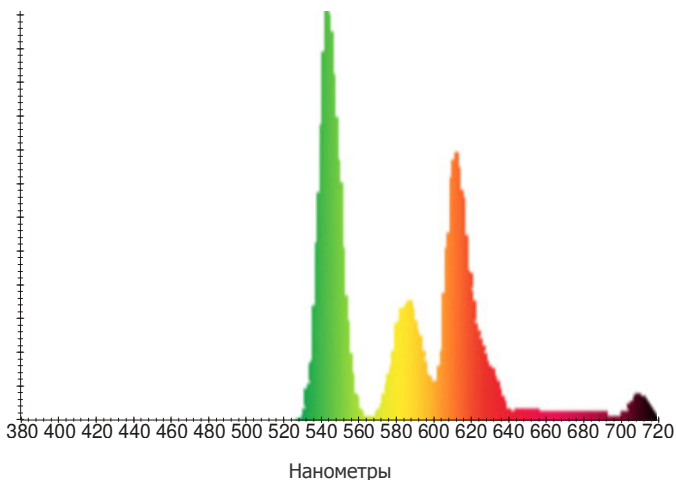
Спектральное распределение
